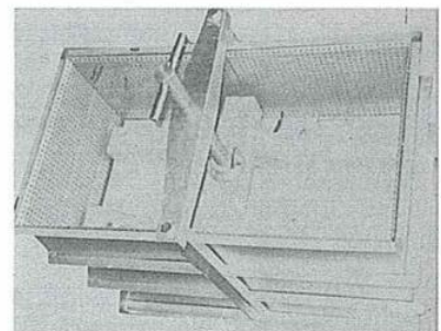
手廻式吟醸搾り機
